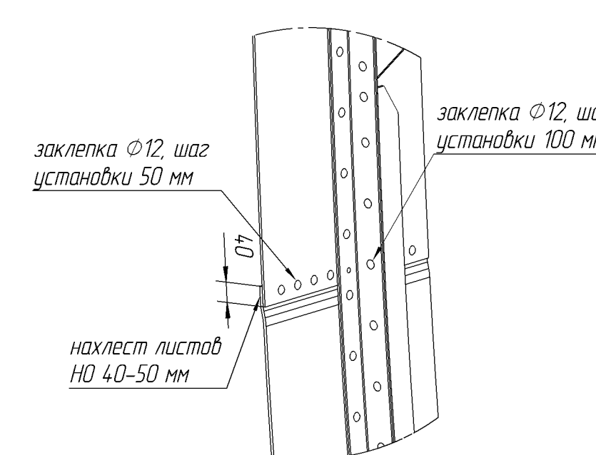
Вид Е
