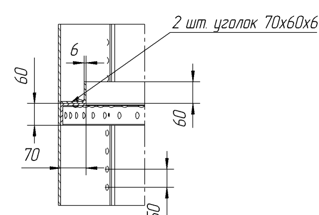
Сечение Б-Б
