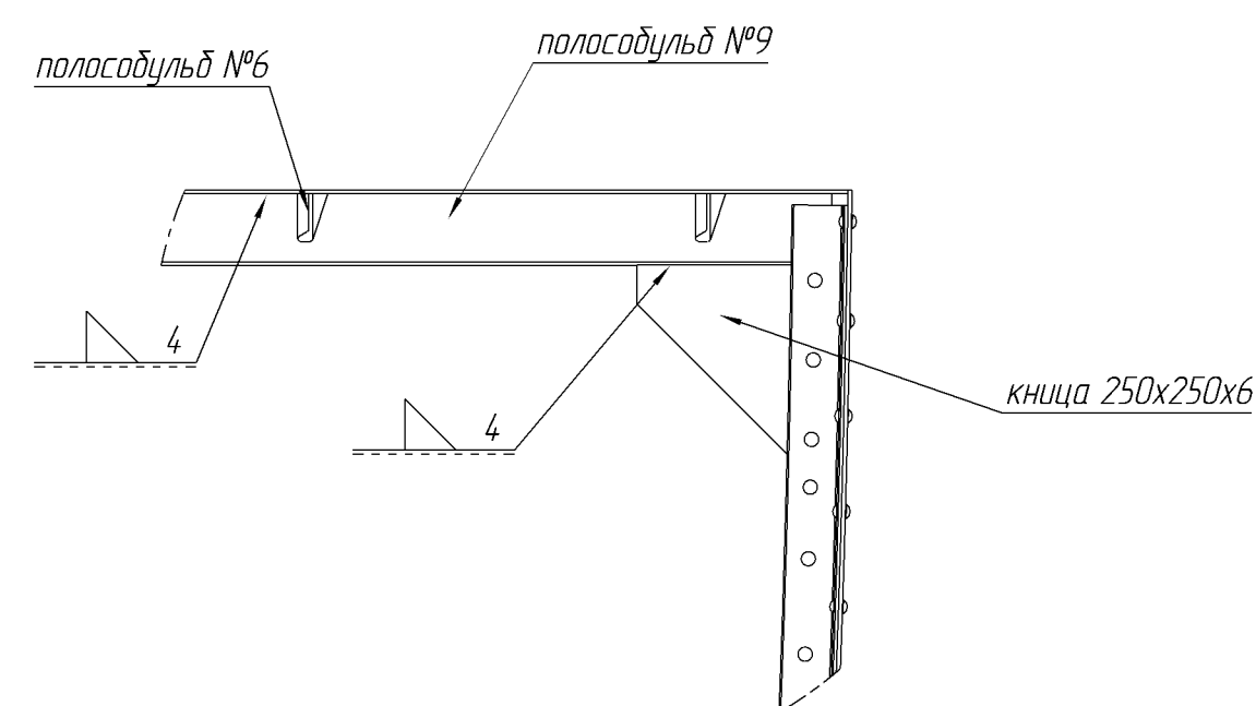
Вид А
