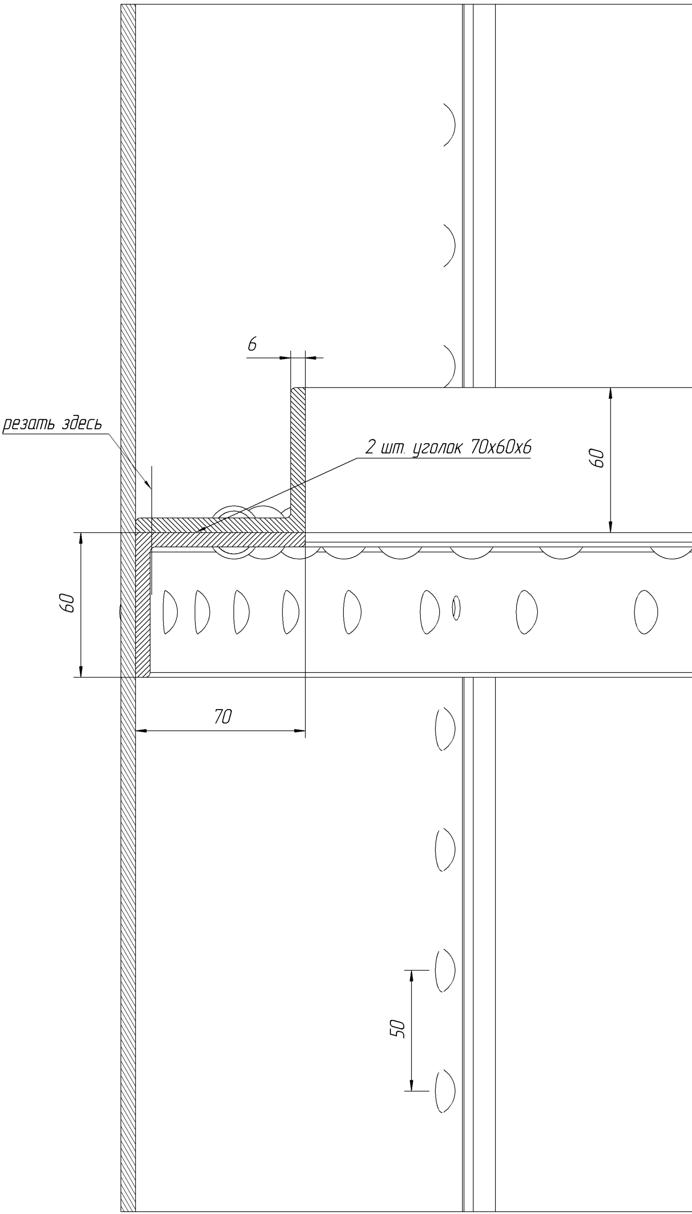
Исходное поперечное сечение бортового набора
