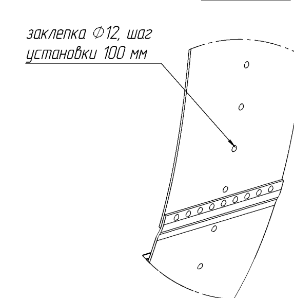
Вид Ж
