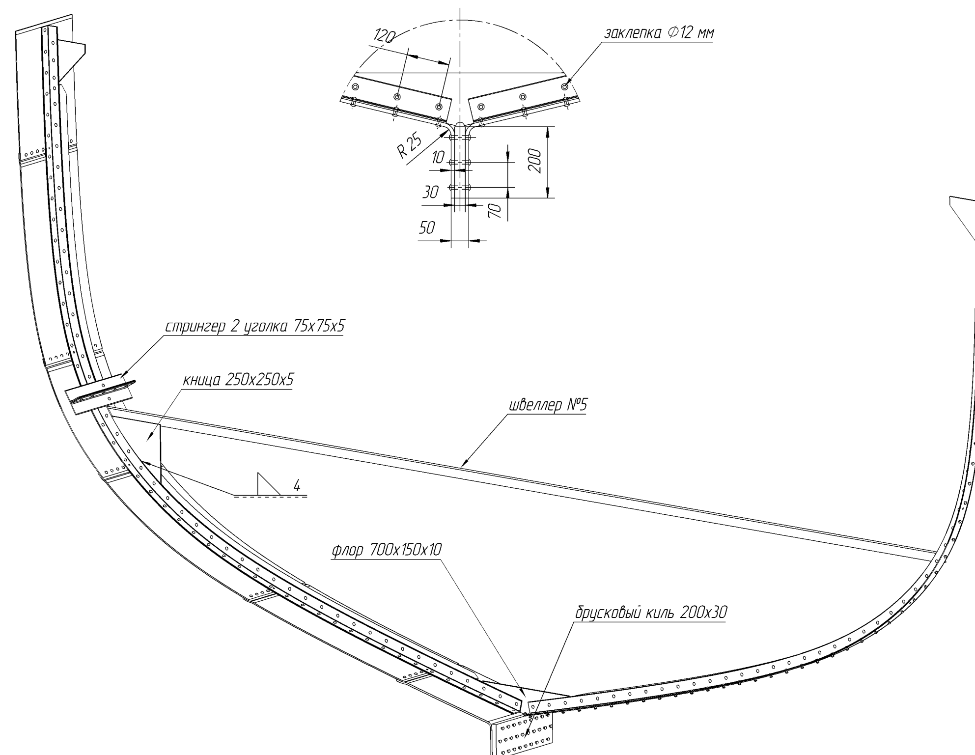
Вид В
