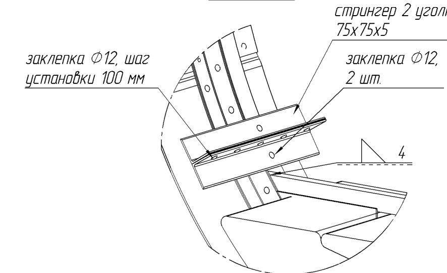
Вид Д
